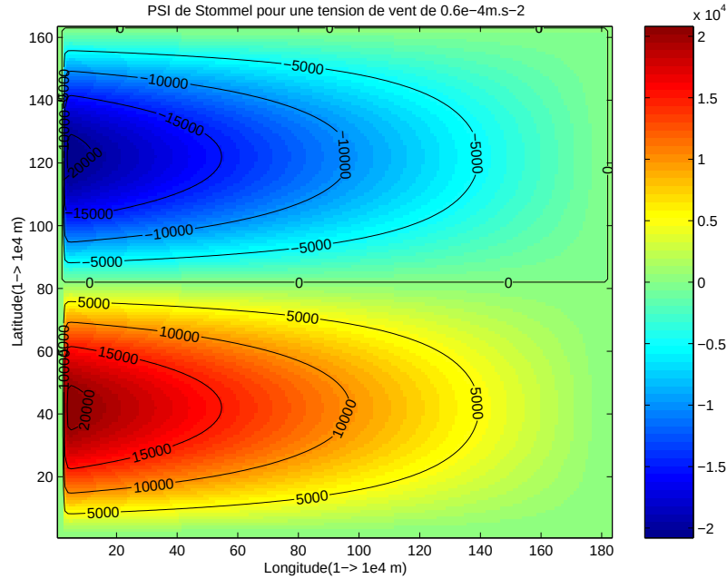
Figure 1: Représentation de la solution linéaire stationnaire, la solution de Stommel: nous observons une intensification de la fonction courant ( \psi en m^2.s^{-1} ) sur le bord Ouest.
