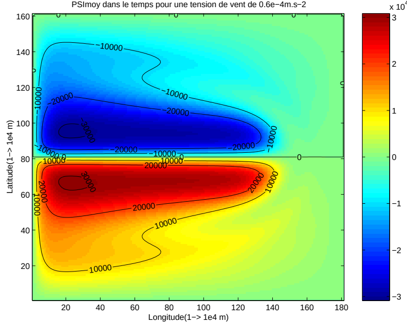
Figure 5: Représentation de la moyenne de la fonction courant \psi en m^2.s^{-1} du modèle numérique prenant en compte la globalité des paramètres. Nous pouvons voir une intensification de \psi au centre du bassin qui n'était pas prévue par la solution de Stommel (figure 1).
