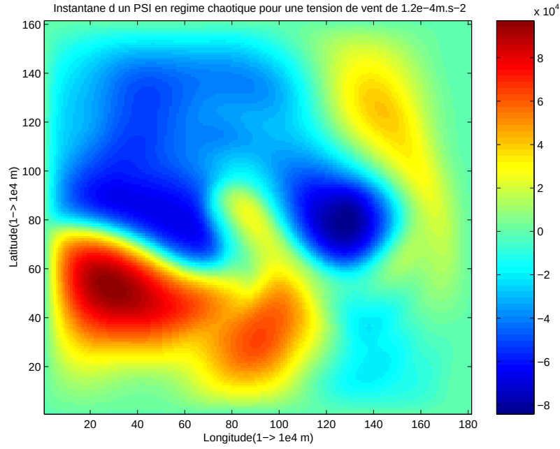
Figure 9: Instantané des modulations dans le bassin, lors du régime apériodique. Nous pouvons voir le franchissement de la ligne neutre et même sa quasi disparition.
