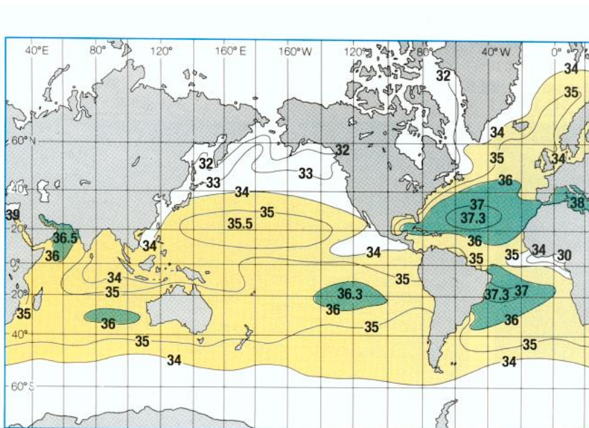
(a) Salinité de surface de l'océan (SSS Sea Surface Salinity)
