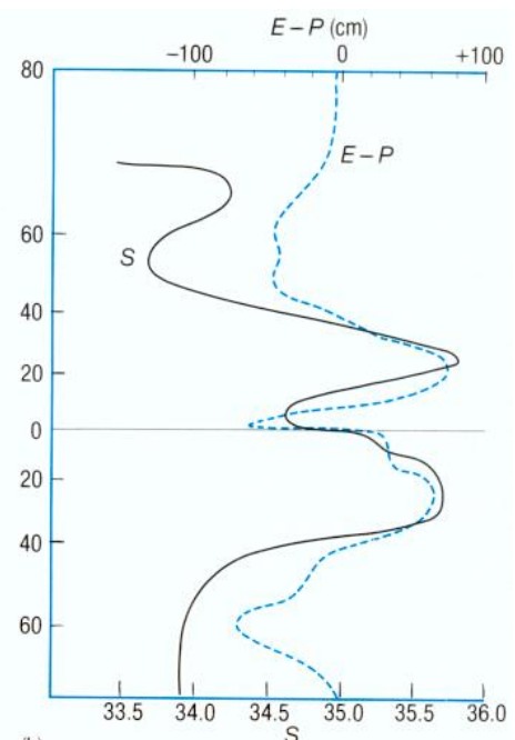
(b) Evaporation - Précipitation
